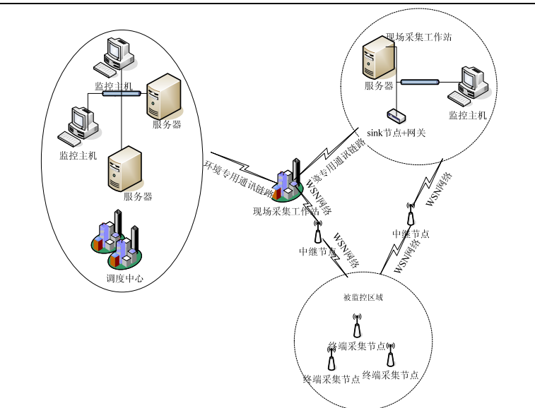
图1 系统结构图
