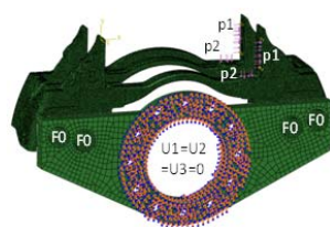
支架优化分析
