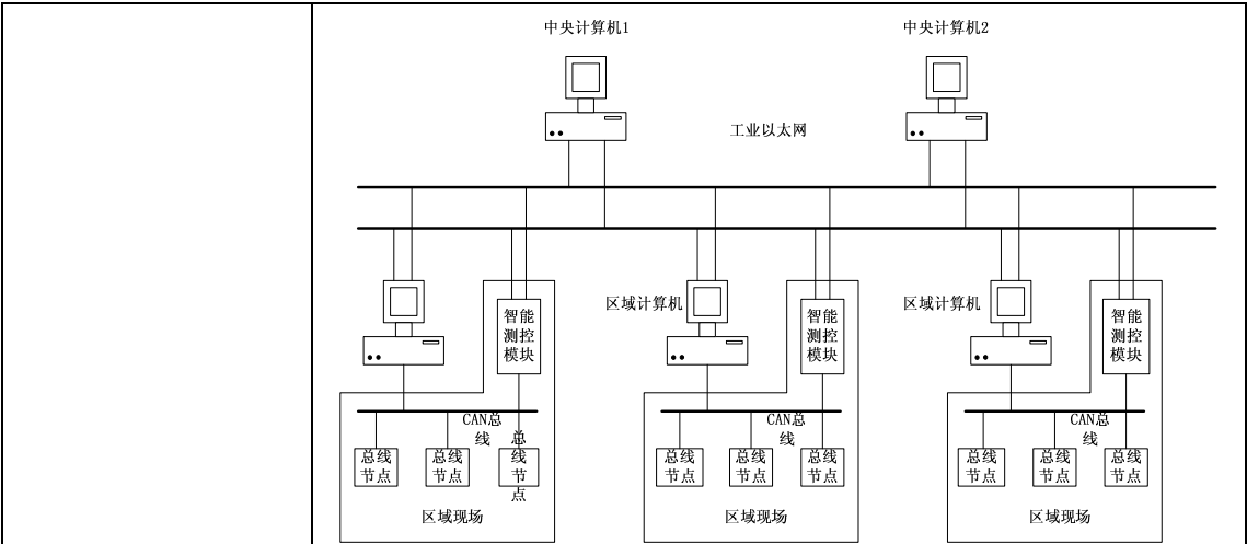
图 2 配电网监控系统示意图
