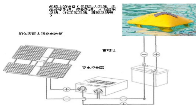
无人水面监测复合三体冲翼艇太阳能系统
