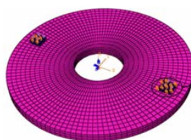
摩擦磨损分析
